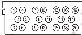
Разъем кабеля Signal/Video in/out
