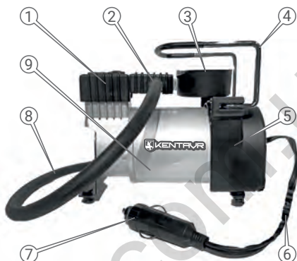
Рисунок 1. Загальний вигляд компресора автомобільного «AK-15035A»
