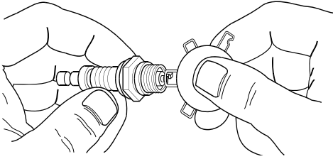
Рис. 6. Проміжок між електродами свічки запалювання
