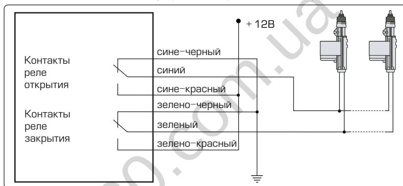
Схема подключения к двухпроводным приводам системы управления
