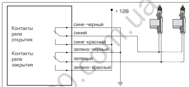
Схема подключения к двухпроводным приводам системы управления
