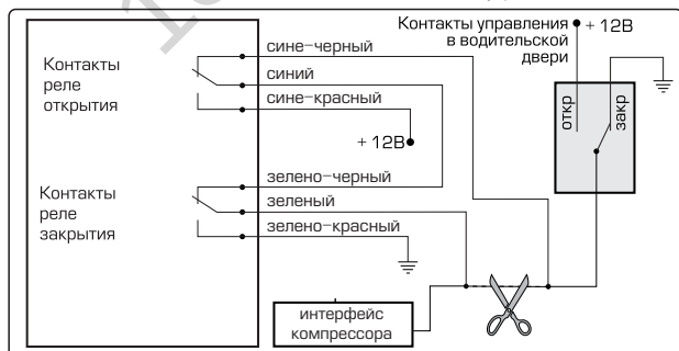
Схема подключения к пневматической системе управления
