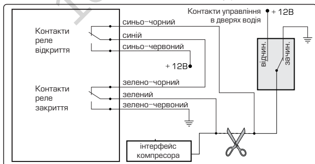
Схема підключення до пневматичної системи управління
