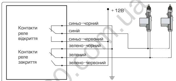
Схема підключення до двохдротовим приводам системи управління
