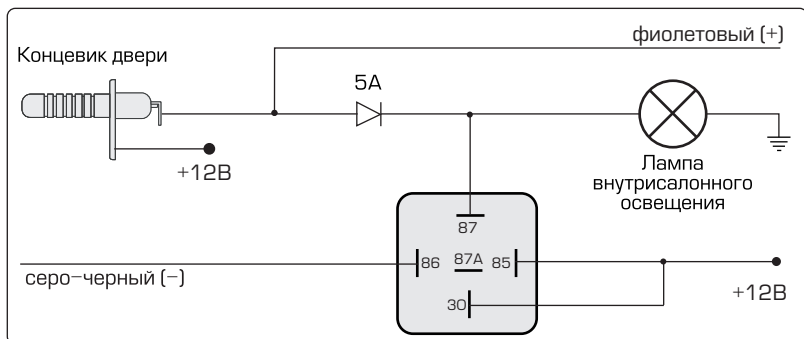
Схема подключения при реализации режимов «Охрана с работающим двигателем» или «Турботаймер»
