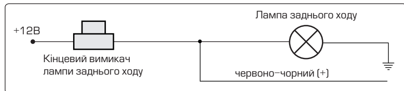
Схема підключення системи для попередження під час руху заднім ходом
