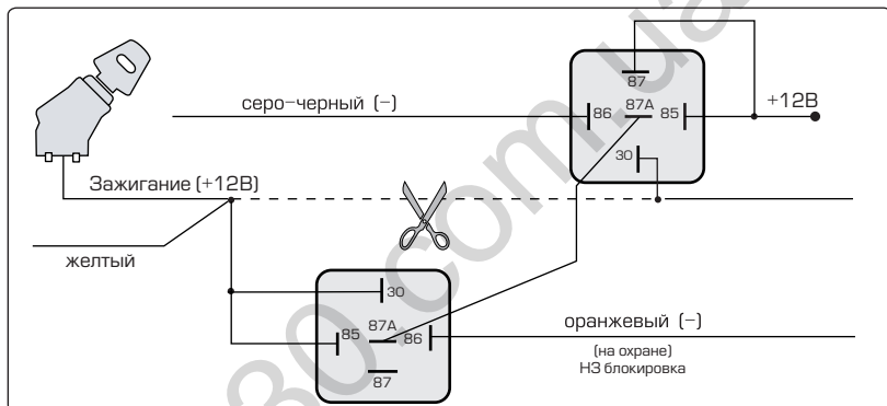
Схема подключения при реализации режимов «Охрана с работающим двигателем» или «Турботаймер»
