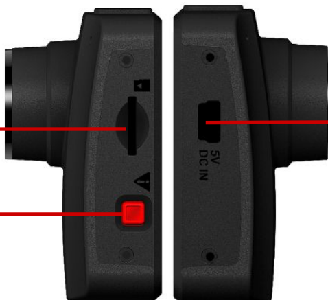
Вигляд збоку
