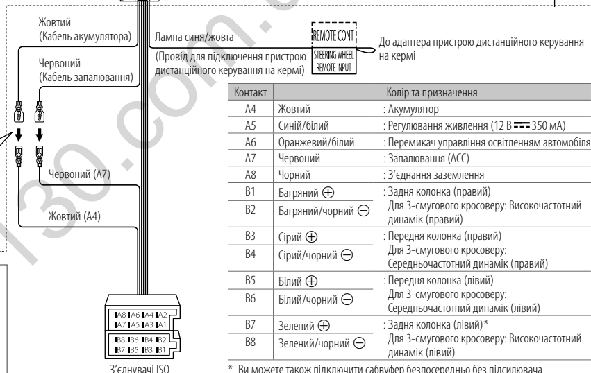
Стандартний варіант схеми підключення проводів
