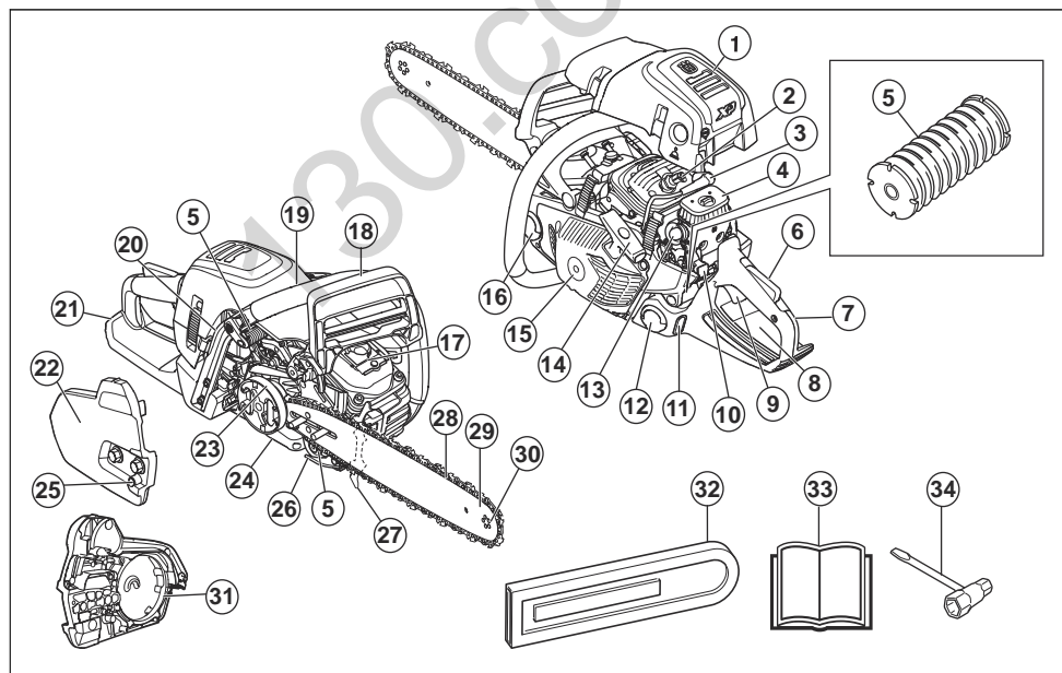
1. Крышка цилиндра
