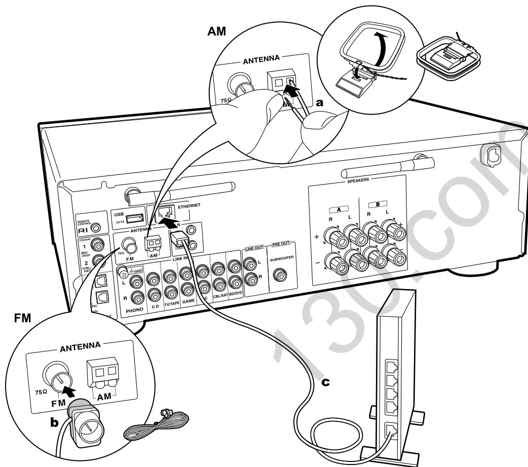
a. Комнатная антенна FM, b. Комнатная антенна AM, c. Кабель Ethernet.
