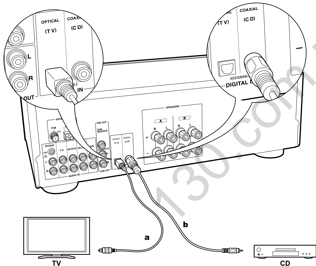
А Цифровой оптический кабель В Цифровой коаксиальный кабель
