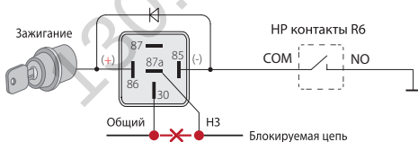
Подключение внешнего реле блокировки
