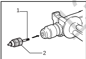
1. Переходник патрона
