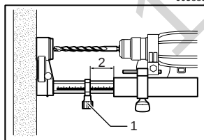
1. Стопор
