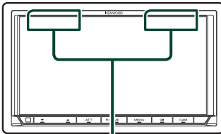
Bluetooth/Wi-Fi-Antenne
