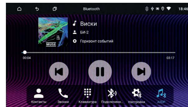
Приложение A2DP
