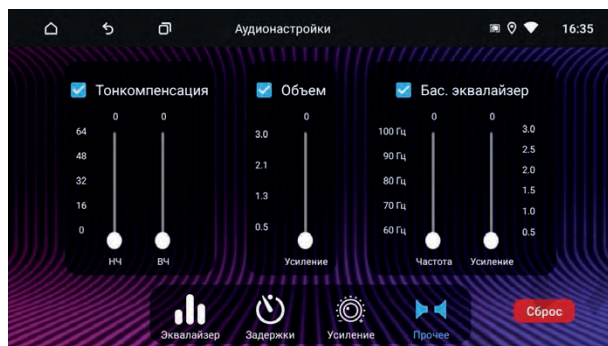
Настройка тонкомпенсации
