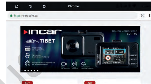
Браузер Chrome
