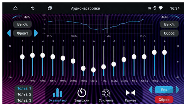
Настройки эквалайзера
