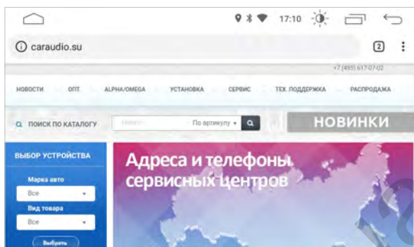
Браузер Chrome
