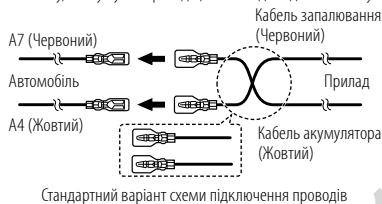
Стандартний варіант схеми підключення проводів
