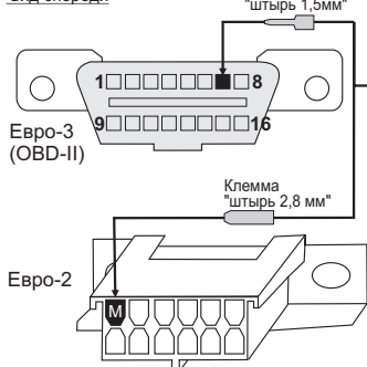
Диагностическая колодка вид спереди
