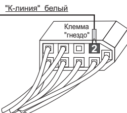
Колодка маршрутного компьютера А/М вид сзади
