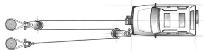
Трехлинейная схема
