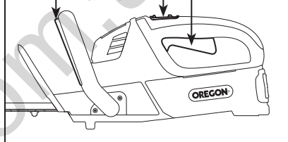
РИС. 15 (3) ВЫКЛЮЧАТЕЛЬ ПИТАНИЯ НА ПЕРЕДНЕЙ РУКОЯТКЕ (2) РЕГУЛЯТОР СКОРОСТИ (1) ПРЕДОХРАНИТЕЛЬ РЕГУЛЯТОРА
