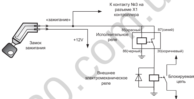
Рис. 10. Подключение реле RDU®, RDD® при блокировке силовоточных цепей с помощью внешнего электромеханического реле. Подключение реле RDUK® при блокировке силовоточных цепей, информационных цепей, а также цепей питания катушек «зажигания». В скобках указаны цвета проводов реле RDUK®.
