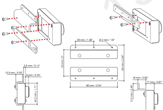
Крепление пульта DRC (опция)
