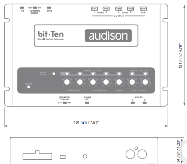
Внешние габариты
