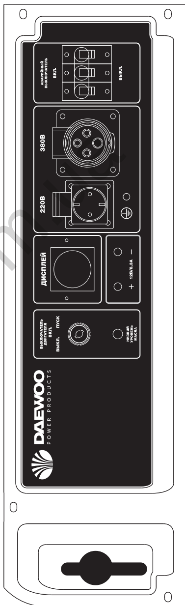
ПАНЕЛЬ ГЕНЕРАТОРА З ЕЛЕКТРОЗАПУСКОМ
