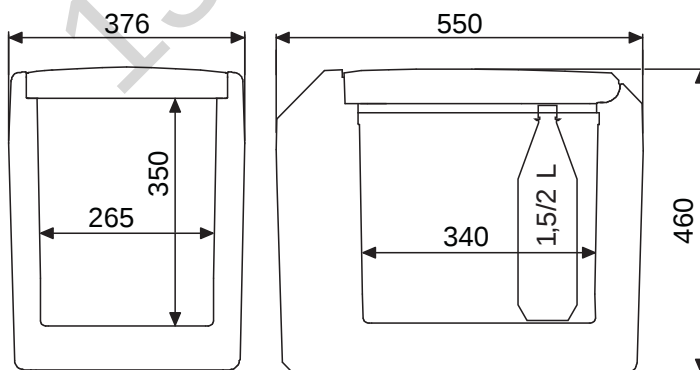
TC35FL-AC
