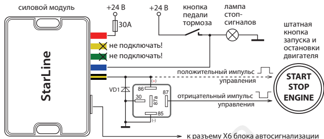
Схема 2: слаботочное управление кнопкой «старт-стоп»
