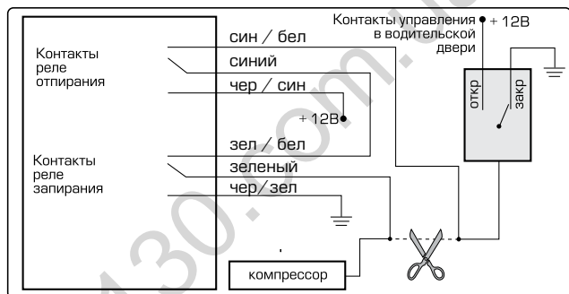
Схема подключения к пневматической системе запирания
