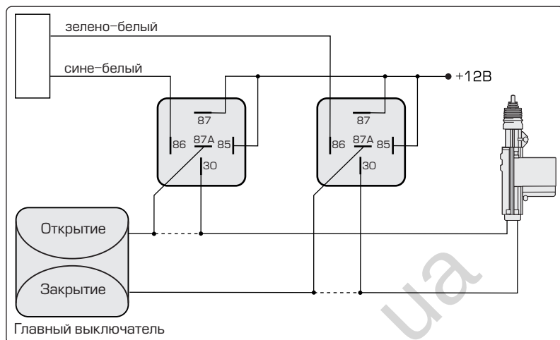
Подключение дверного замка с изменяемой полярностью
