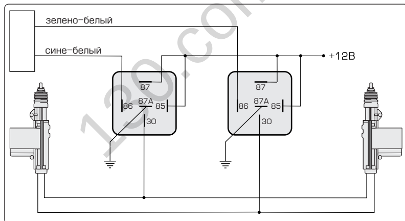
Подключение дополнительного электропривода дверного замка
