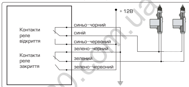
Схема підключення до дводротовим приводам системи управління
