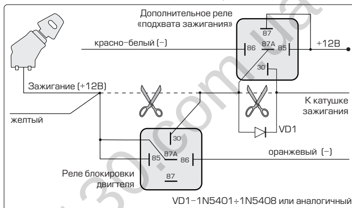
Схема подключения режима «Турботаймер»
