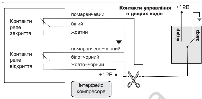
Схема підключення системи до пневматичного ЦЗ
