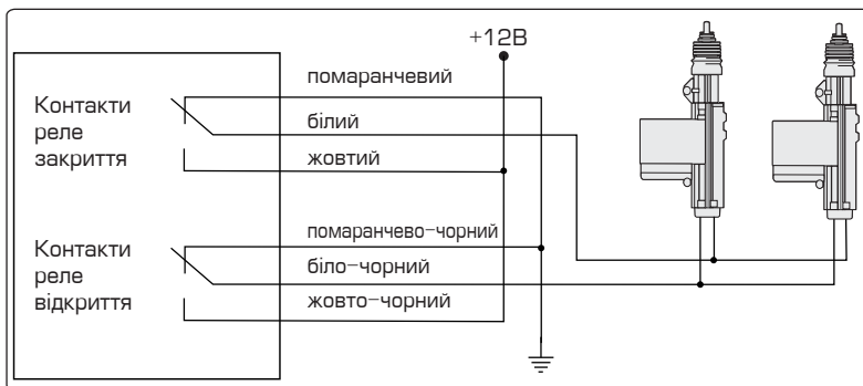
Схема підключення до двопроводних приводів ЦЗ
