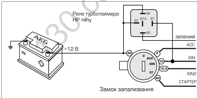
Схема підключення режиму «Турботаймер»
