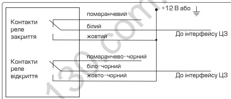
Схема підключення до двопроводних приводів ЦЗ
