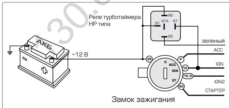
Схема подключения реле «Турботаймера»
