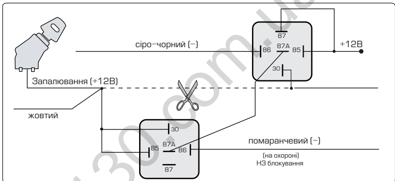
Схема підключення при реалізації режимів «Охорона з працюючим двигуном» або «Турботаймер»
