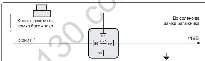
Схема підключення до соленоїда замка багажника з негативною полярністю
