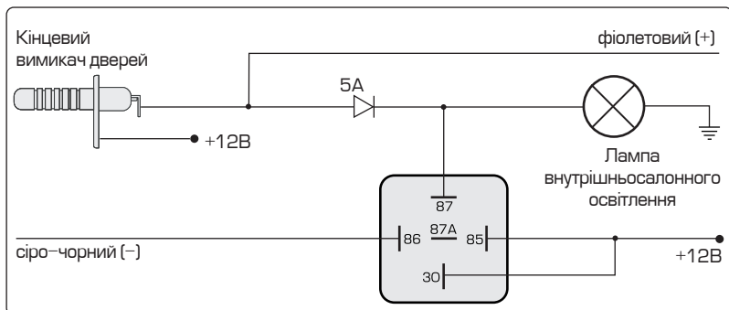
Схема підключення при реалізації режимів «Охорона з працюючим двигуном» або «Турботаймер»
