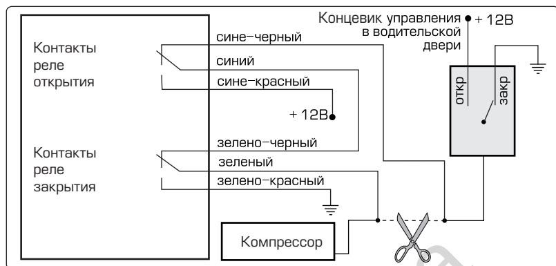
Схема подключения к пневматической системе управления ЦЗ
