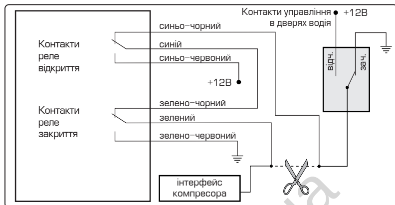
Схема підключення до пневматичної системи управління ЦЗ
