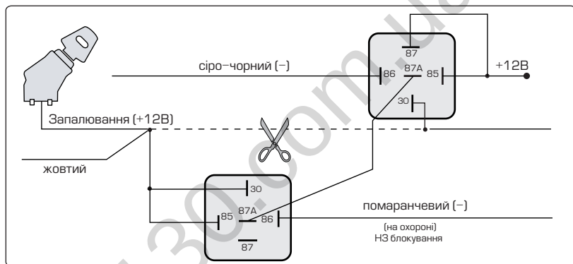
Схема підключення при реалізації режимів «Охорона з працюючим двигуном» або «Турботаймер»
