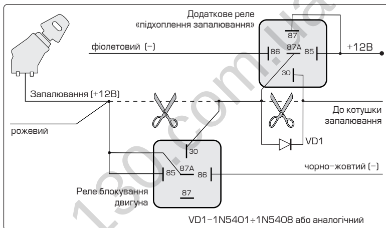
Схема під'єднання режиму «Турботаймер»
