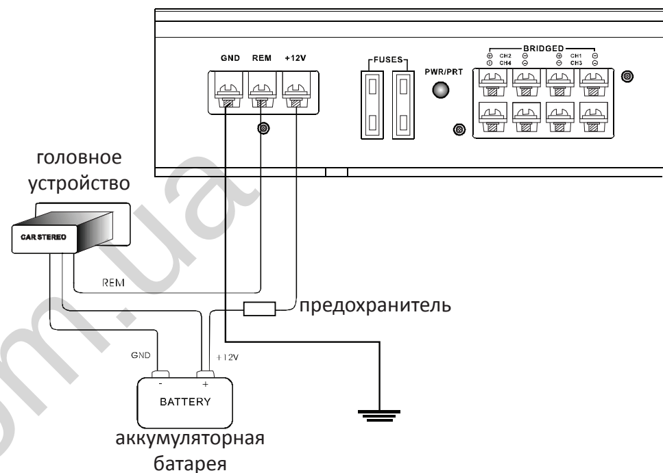
Схема подключения кабелей питания и управления
