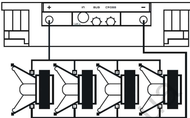
4 динамика 4ohms 2000w Rms Соединены параллельно
