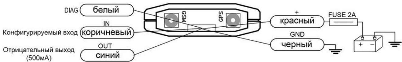
Расположение выводов модуля
