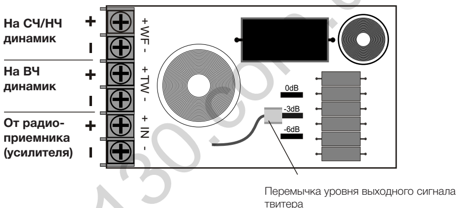
Рисунок 6 Схема подключения кроссовера
