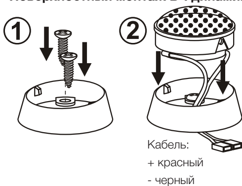
Рисунок 4 Поверхностный монтаж ВЧ динамика
