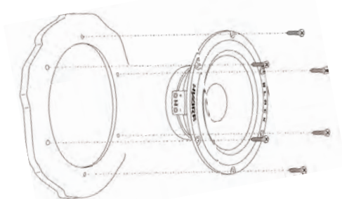
Установка низкочастотного динамика с сеткой гриль
