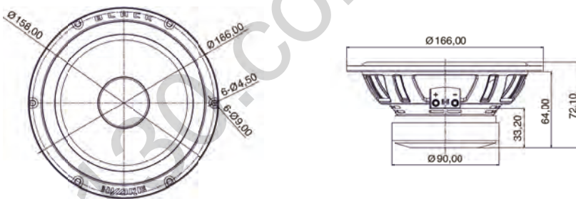
Низкочастотный динамик HDC-2.23W
