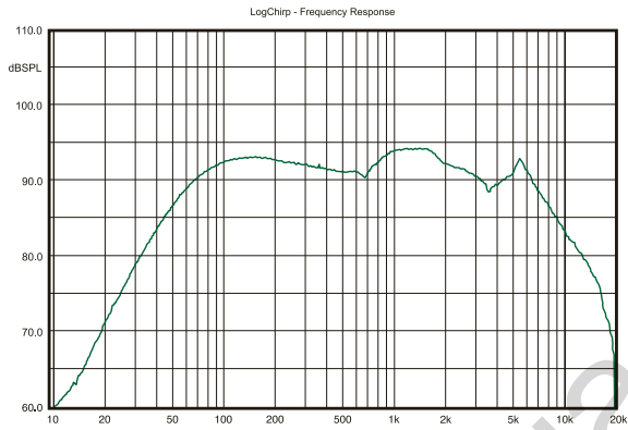
Tweeter HDC-2.23T
