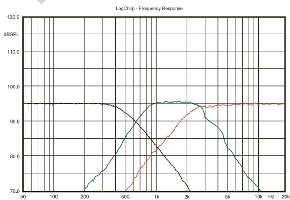
Кроссовер HDC-2.23С
