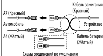
Схема соединений по умолчанию
