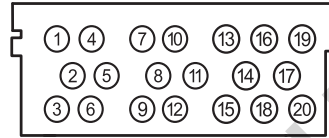
Роз'єм для підключення кабелю Signal / Video in / out
