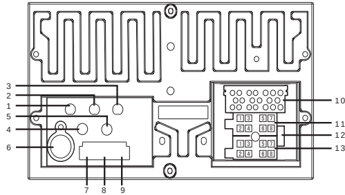
Роз'єм для підключення кабелю Signal / Video in / out
