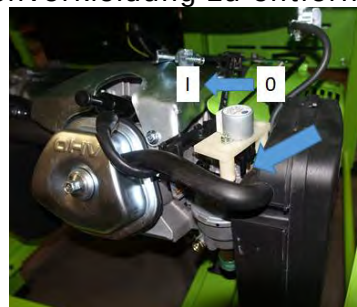
Drosselklappe Pos. 0 für Startvorgang. Pos. I im Betrieb.
