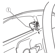
1 Doppelseitiges Klebeband
