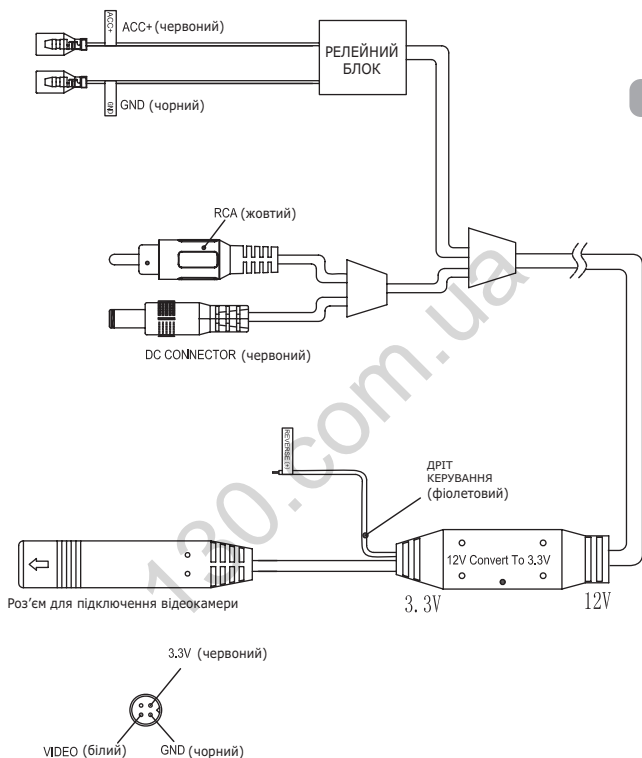
Схема блоку комутації та управління Gazer AC100
