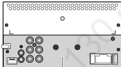
Achterzijde van het toestel
