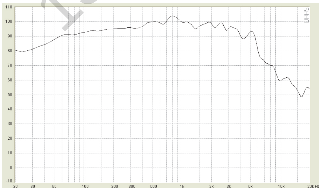
FREQUENZGANG AUF ACHSE / FREQUENCY RESPONSE ON AXIS
