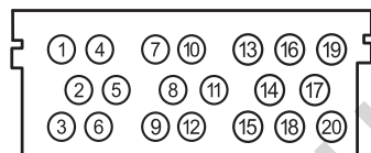
Роз'єм для підключення кабелю Signal/Video in/out
