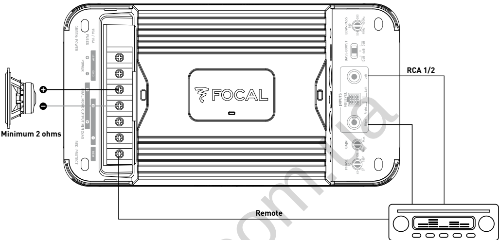
fig. 3.3 - FD 1.350, connexion simple bobine
