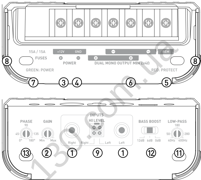
fig. 7.3, FD 1.350
