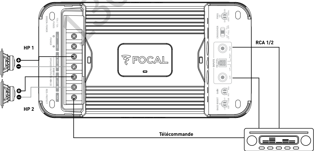
fig. 3.2 - FD 2.350
