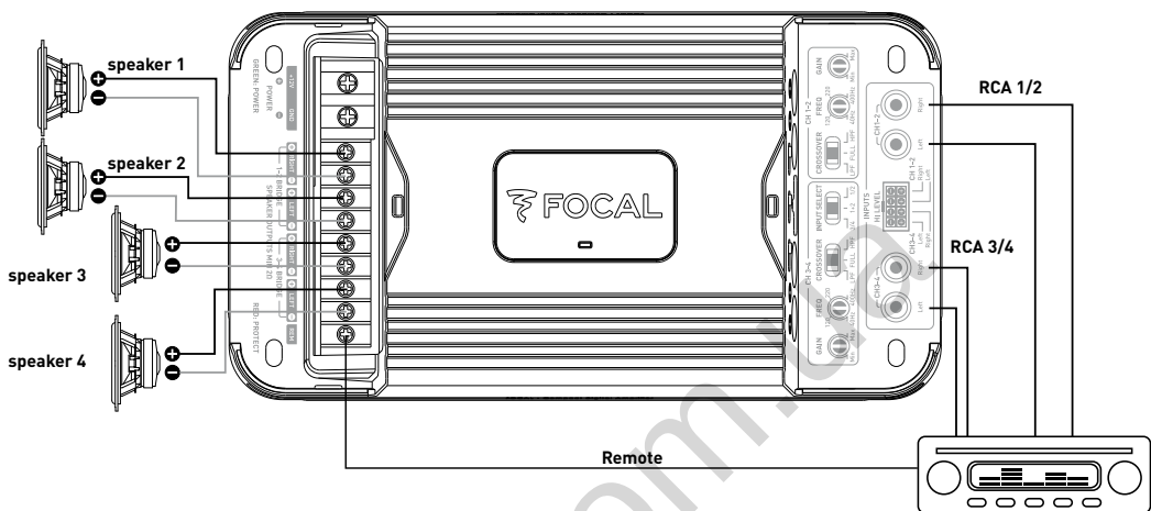
fig. 3.1 - FD 4.350
