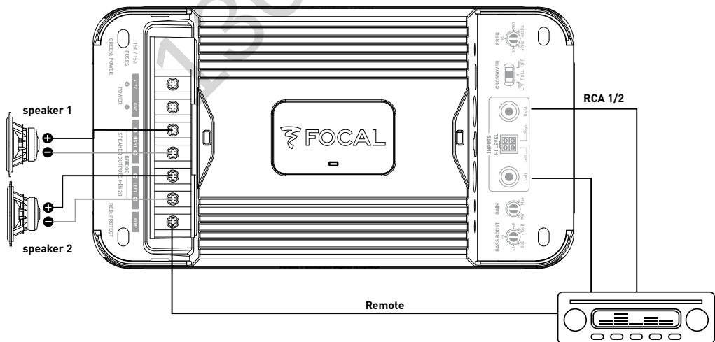
fig. 3.2 - FD 2.350
