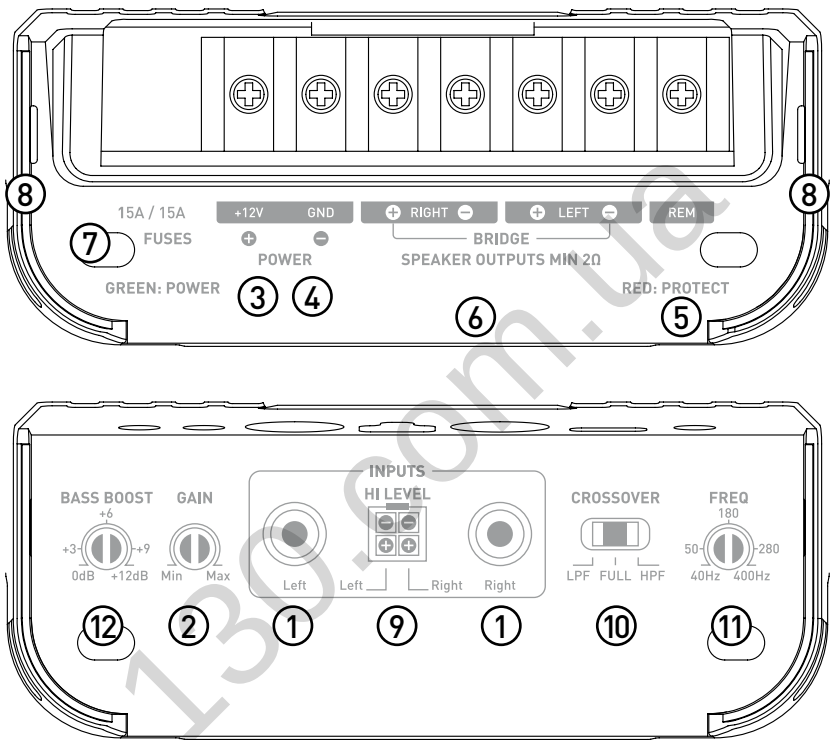
fig. 7.2, FD 2.350
