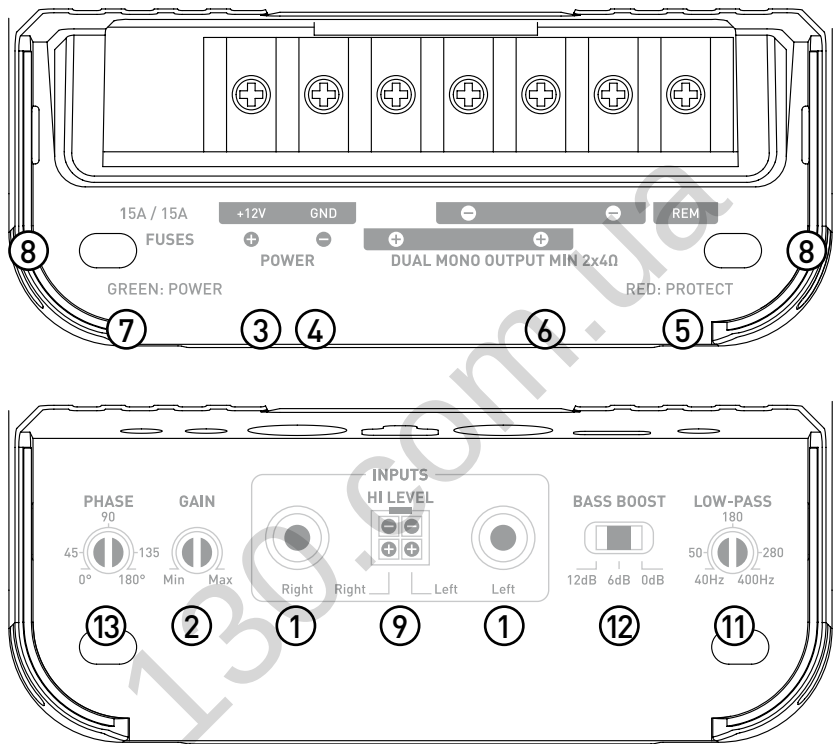
fig. 7.3, FD 1.350
