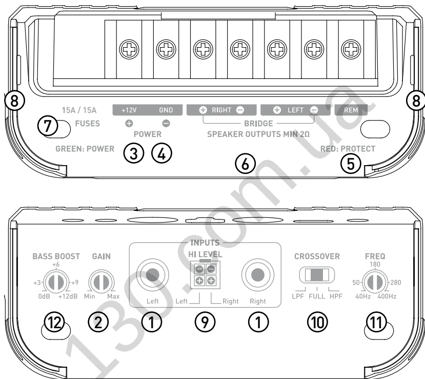
fig. 7.2, FD 2.350
