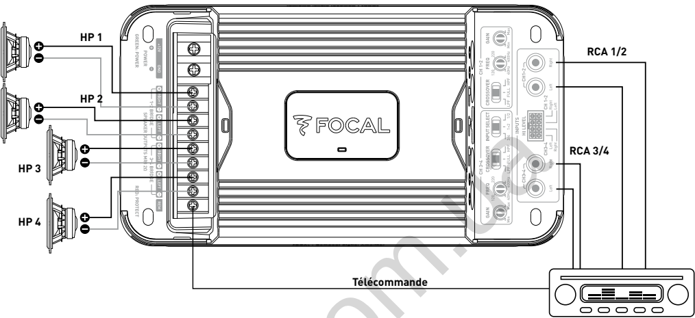
fig. 3.1 - FD 4.350
