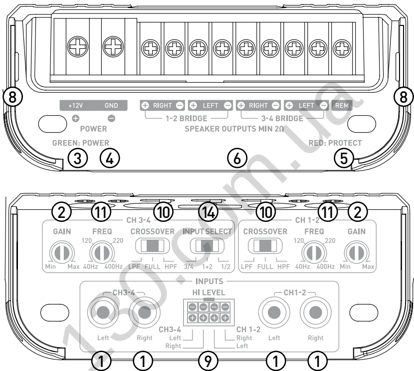
fig. 7.1, FD 4.350
