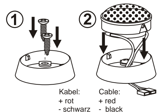
Abbildung 4 Aufbau Hochtöner Figure 4 Surface mount of Tweeter
