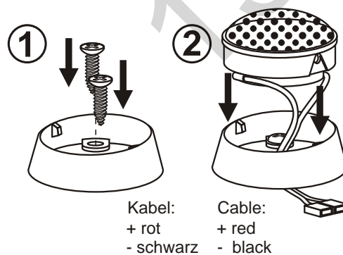
Abbildung 4 Aufbau Hochtöner Figure 4 Surface mount of Tweeter
