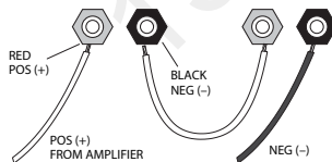
Afbeelding 2. Serieaansluiting
