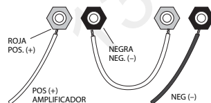
Figura 2. Conexión en serie
