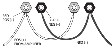
Afbeelding 1. Parallelaansluiting
